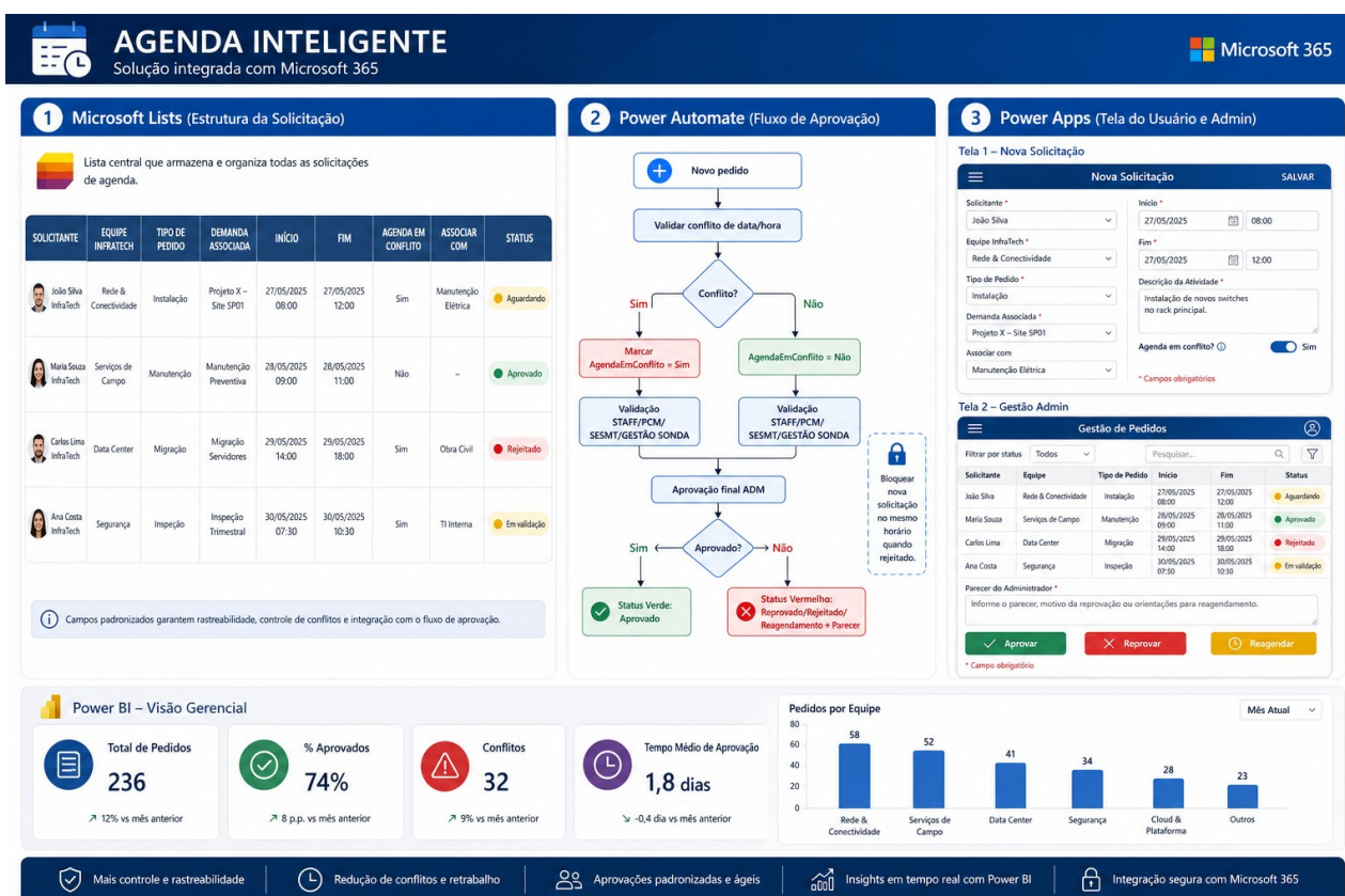
Figura 1 - Arquitetura visual (List + Automate + Power Apps + BI)
